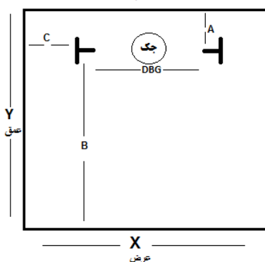
نمای بالا از چاهک
